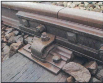
安装普通螺母
