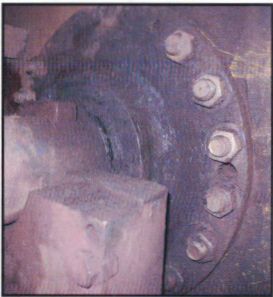
摆式飞轮安装普通螺母
