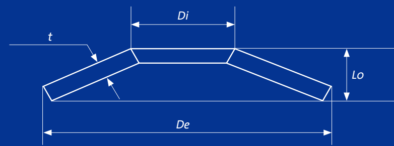
碟形弹簧尺寸参数：
